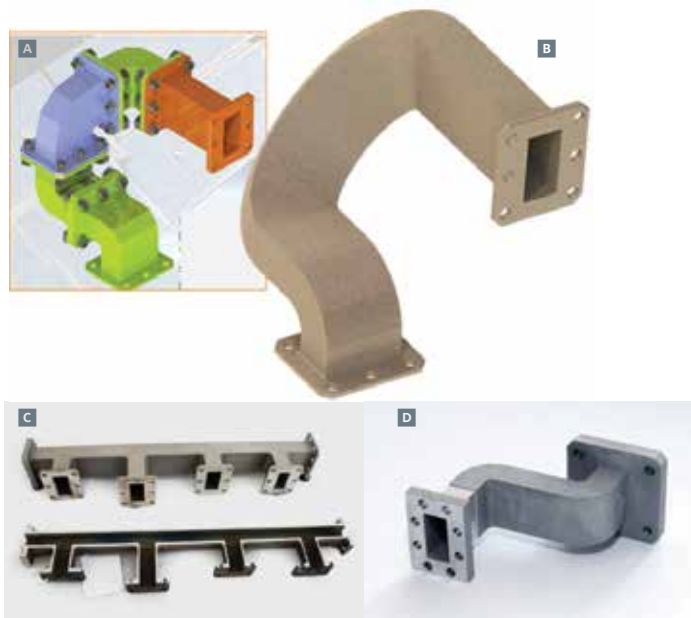
5 Традиционный волновод A ; волноводы, изготовленные 3D-печатью B , C , D . Источник: Optisys
