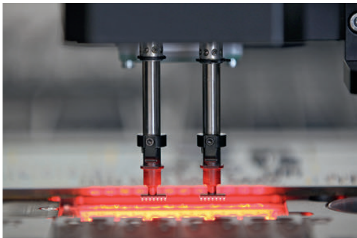
Универсальный сборочный центр Essemtec Fox: универсальные головки для 01005 и 80 x 80 мм
